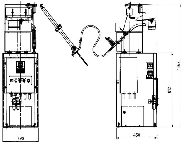
TIPO-VIBRATORIO
