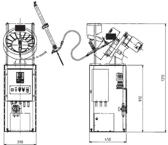
TIPO-ROTATIVO
